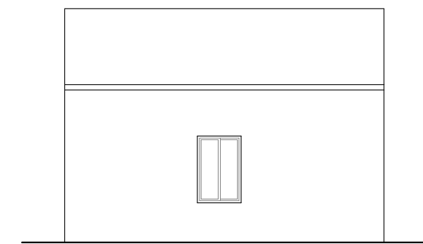
Alzado posterior
